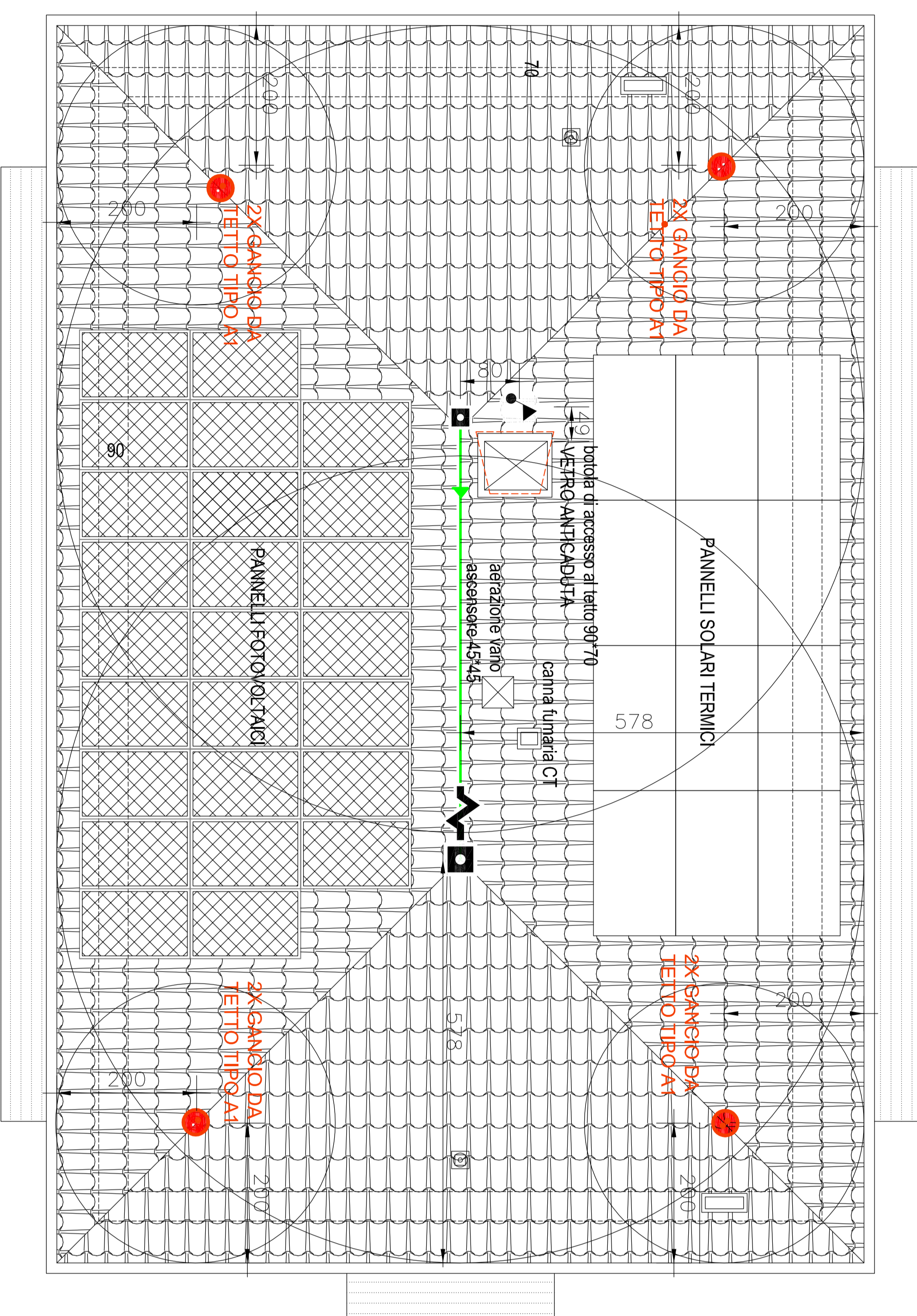
PIANTA COPERTURA 1:50
