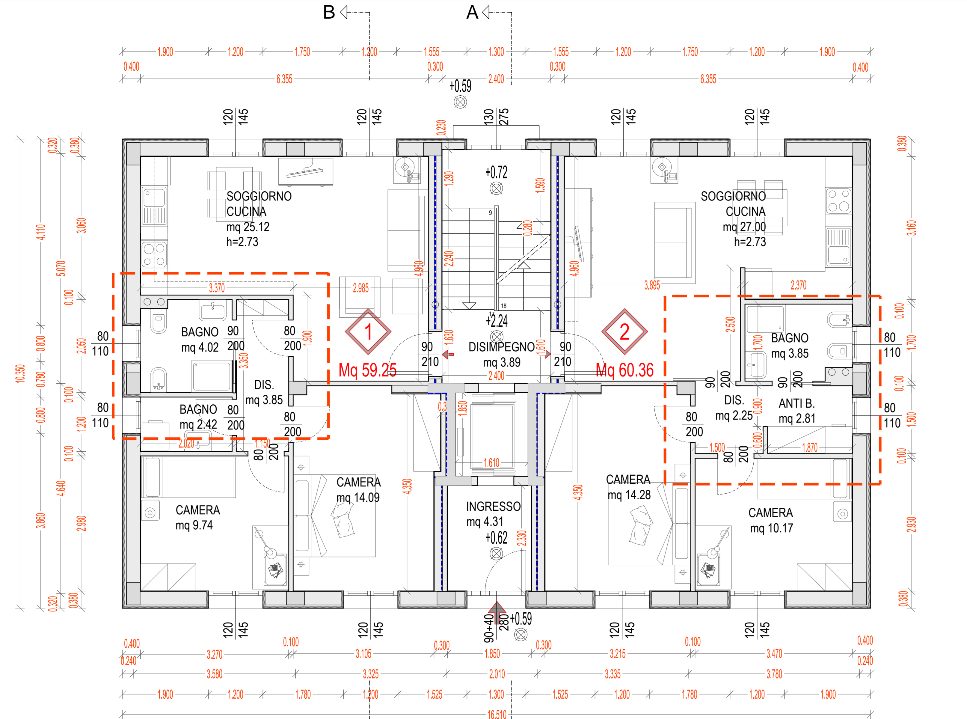
PIANO RIALZATO
