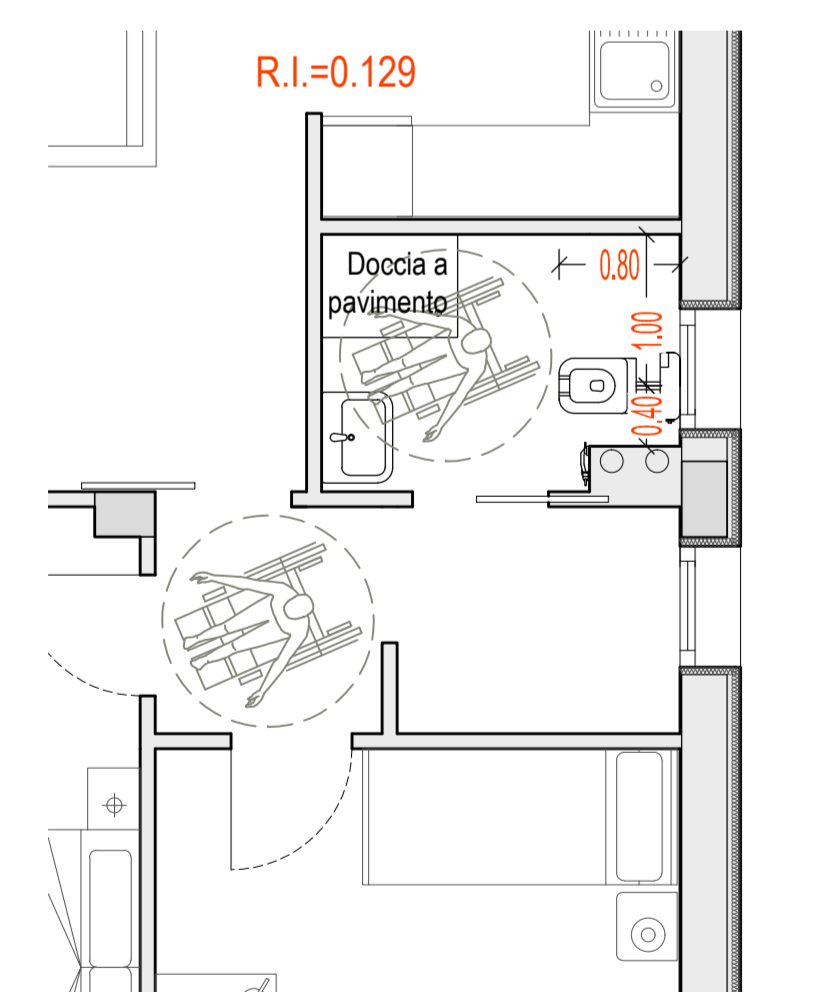
TIPOLOGIA BAGNO APPARTAMENTI 2
