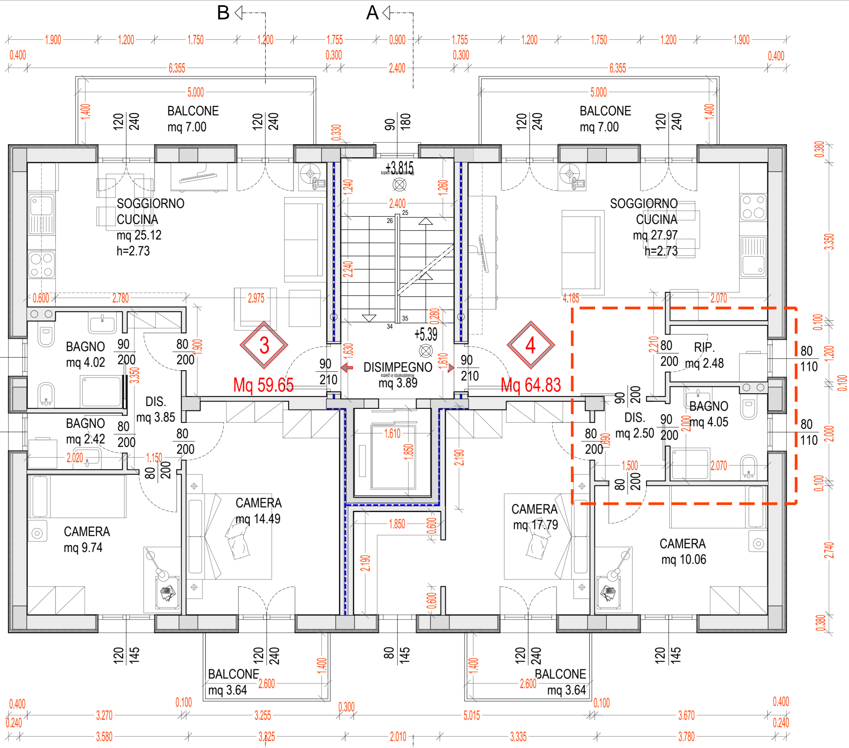
PIANO PRIMO
