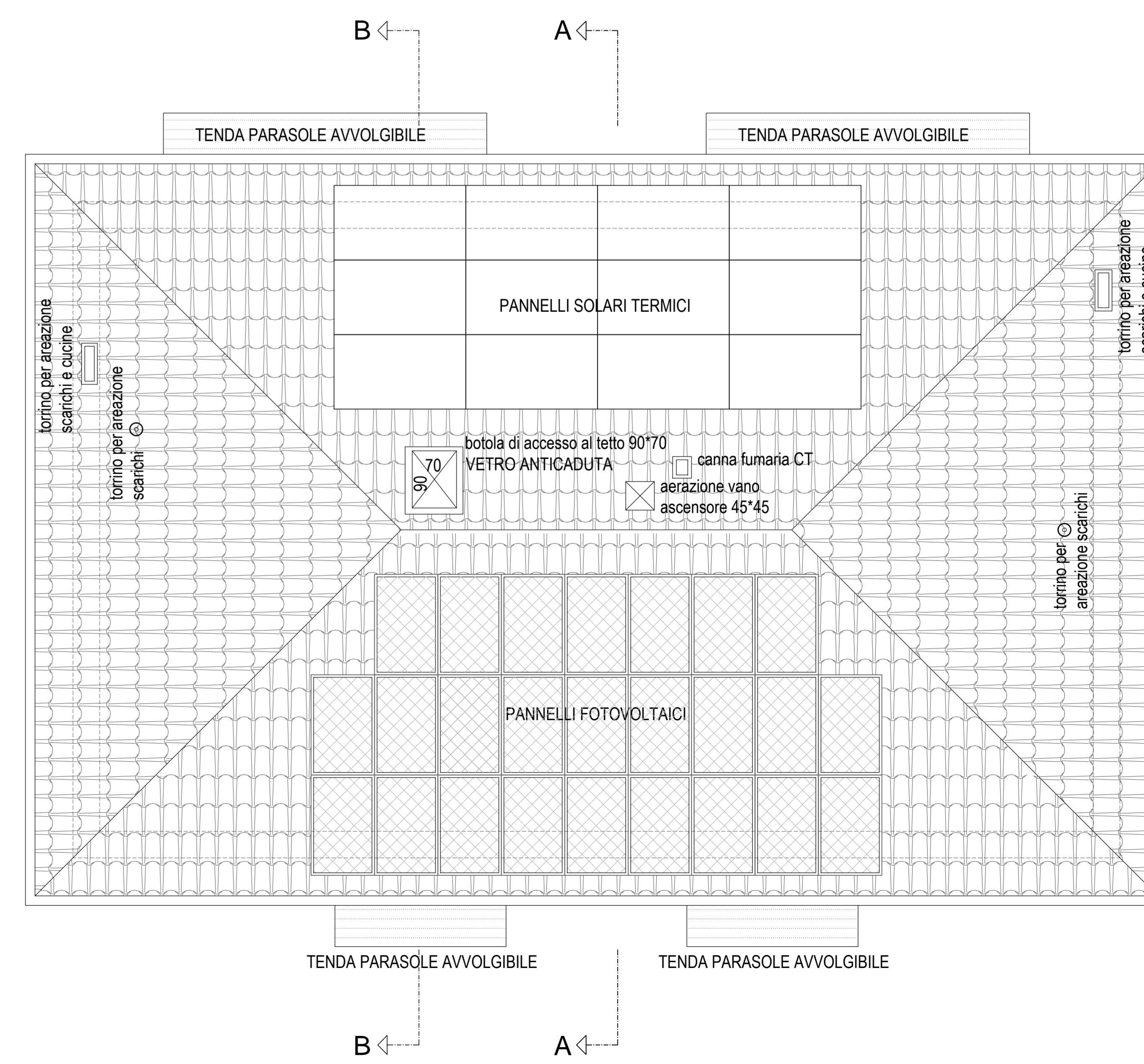
PIANO COPERTURA
