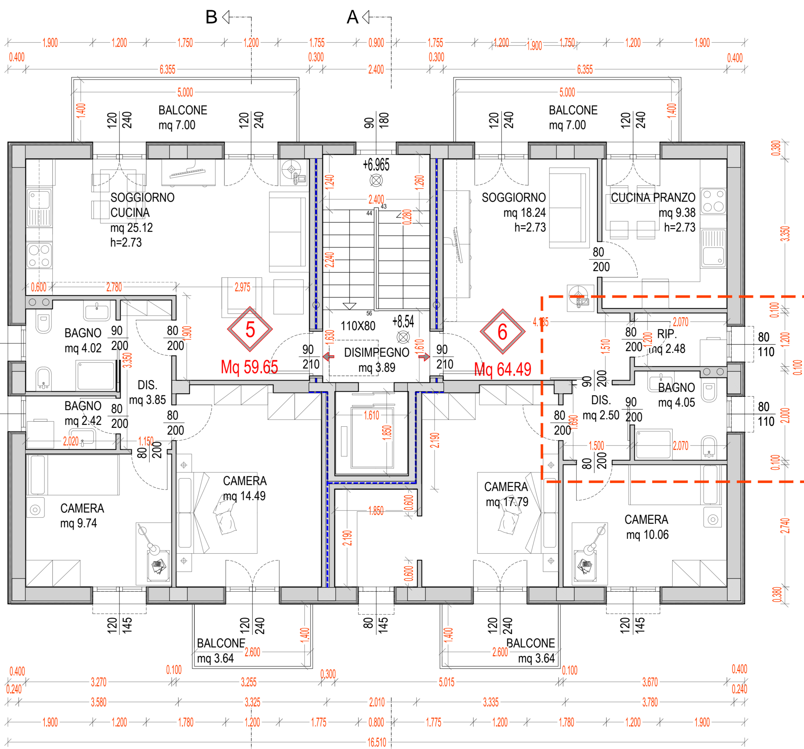
PIANO SECONDO
