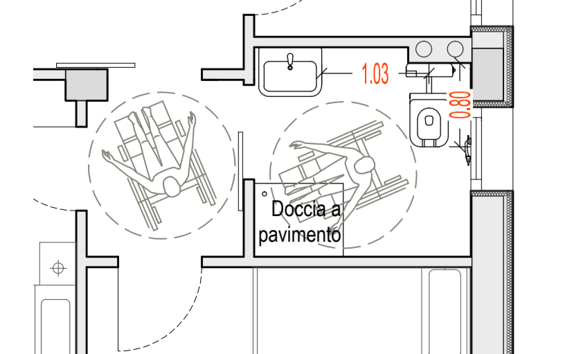
TIPOLOGIA BAGNO APPARTAMENTI 4-6
