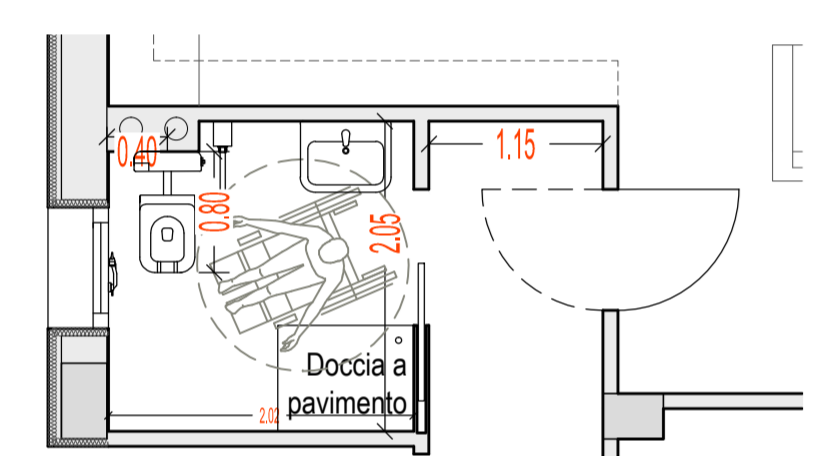
TIPOLOGIA BAGNO APPARTAMENTI 1-3-5
