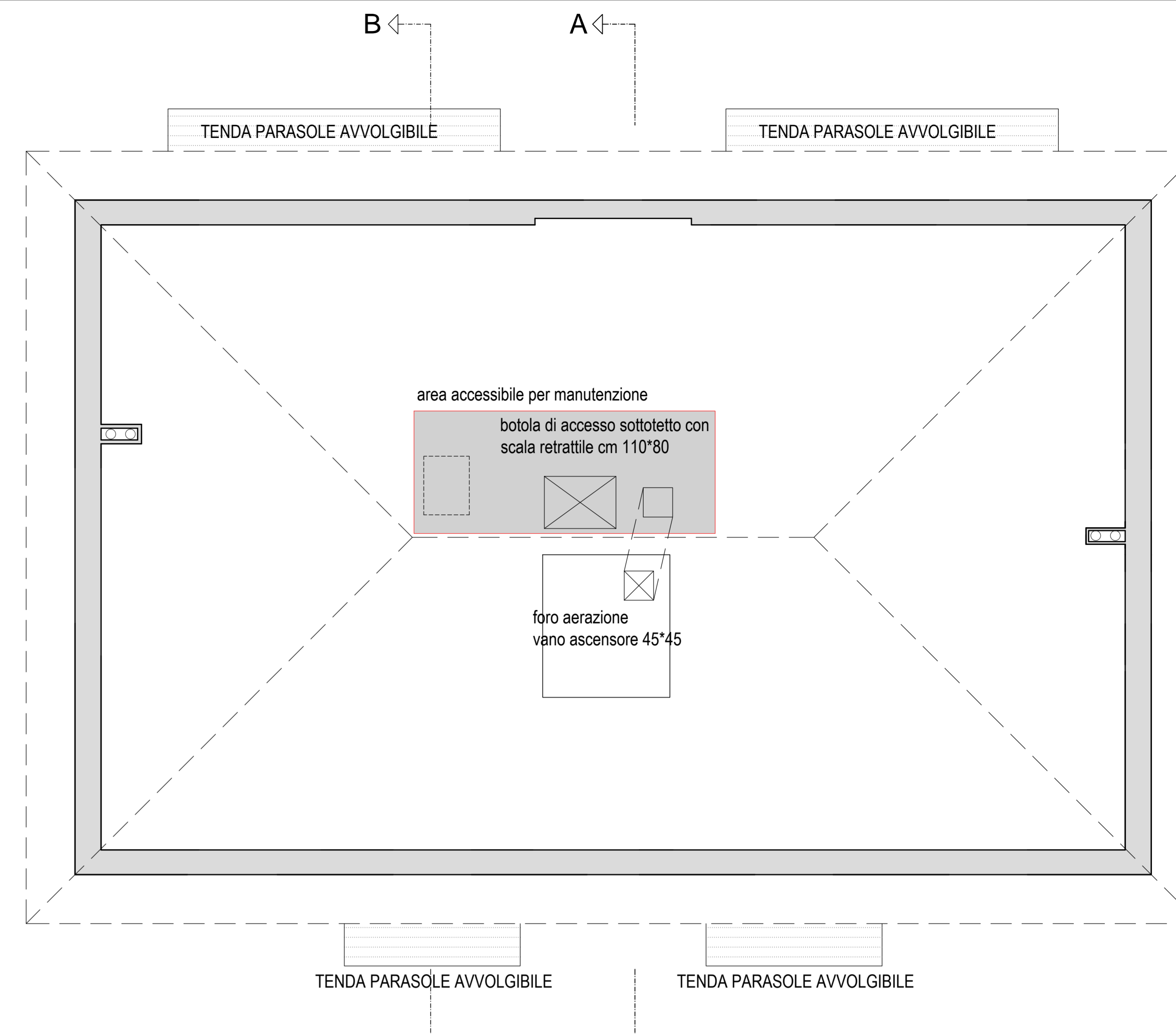
PIANO SOTTOTETTO
