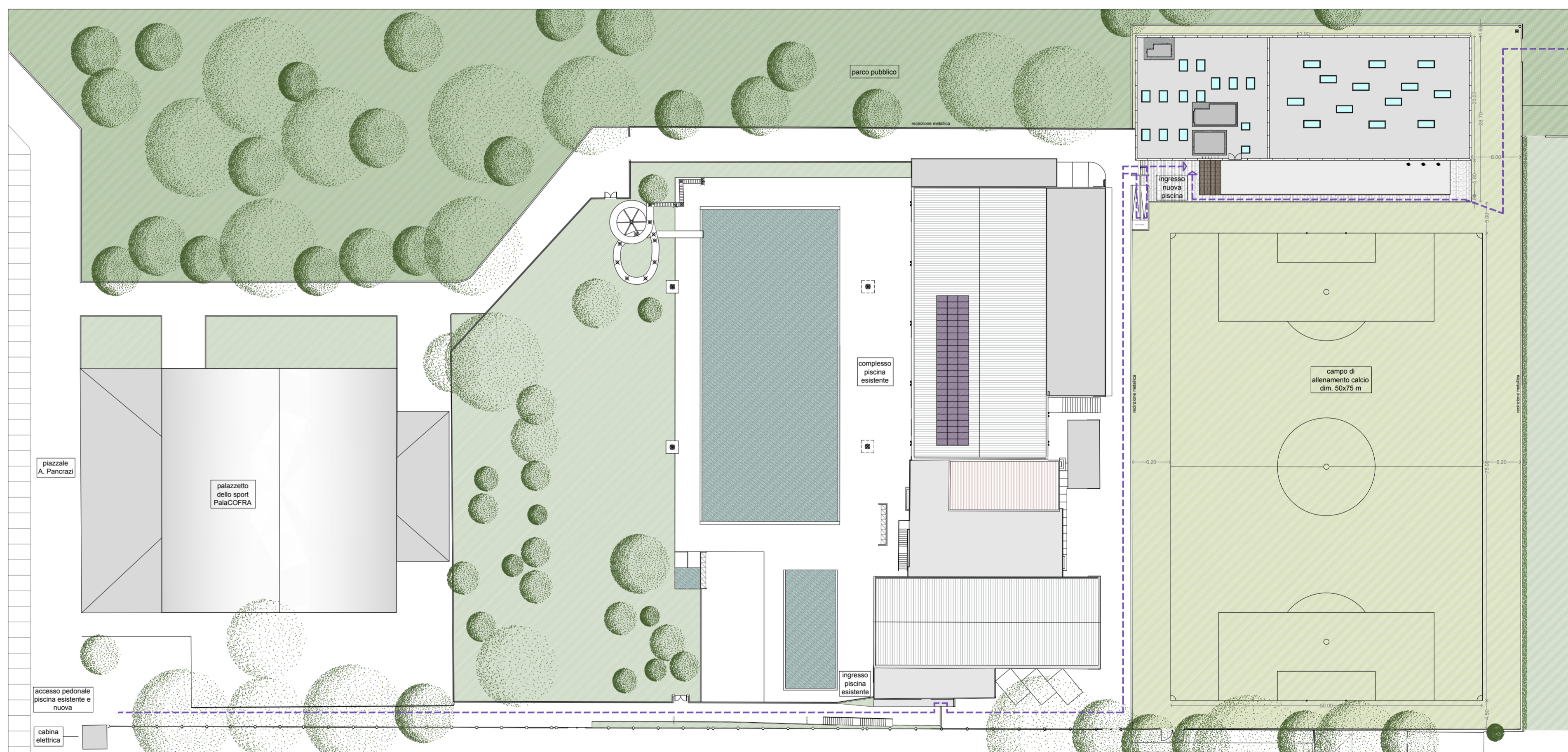
PLANIMETRIA PROGETTO scala 1:500
