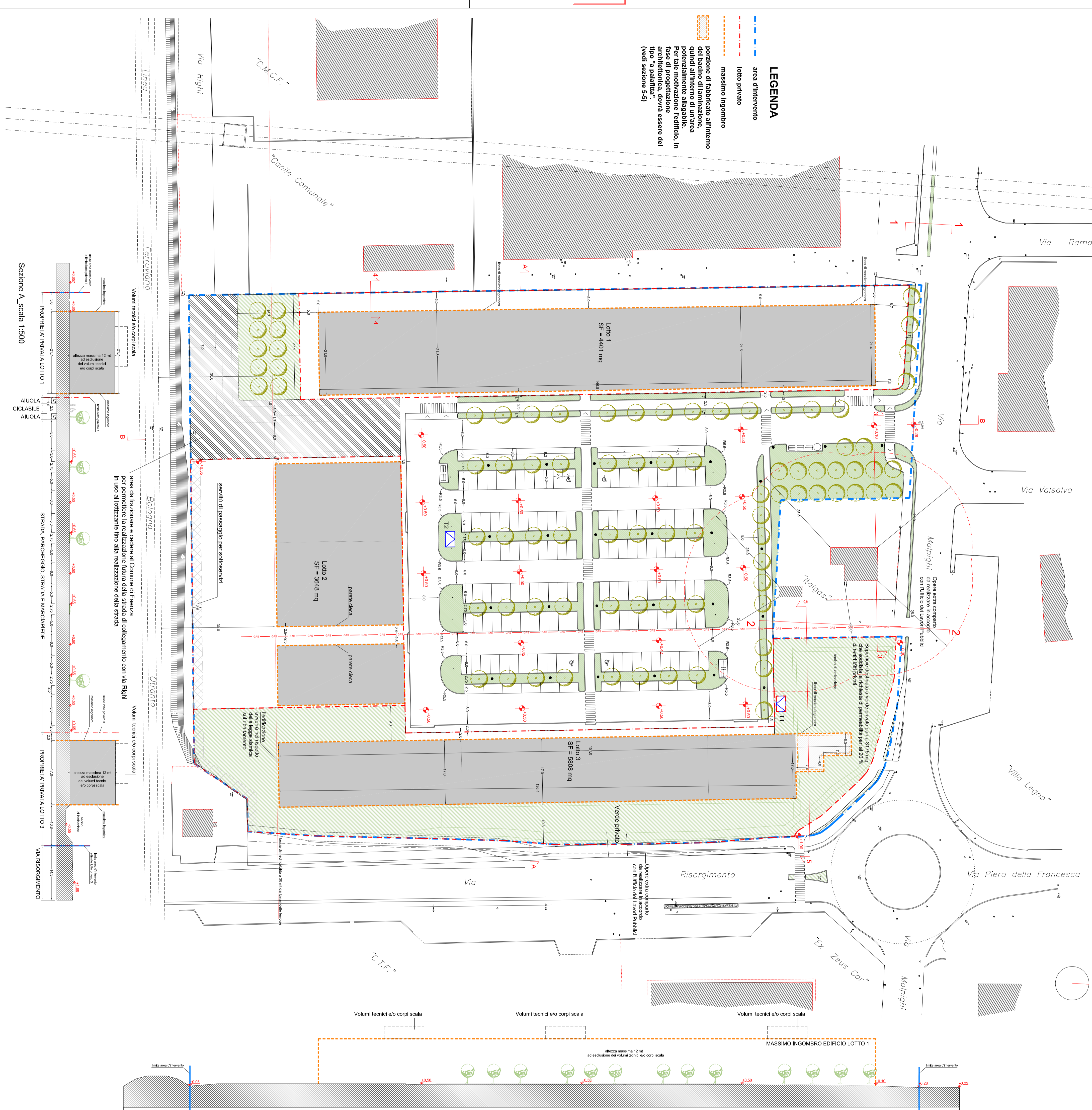
Planimetria architettonica scala 1:500
